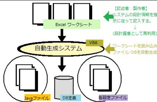
図 1 自動生成システムの全体図
