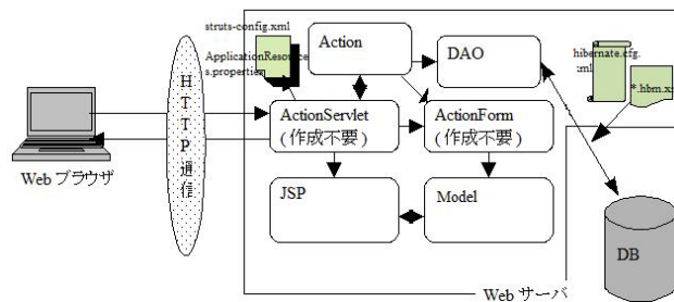
図 2 生成されるアプリケーションの構成
